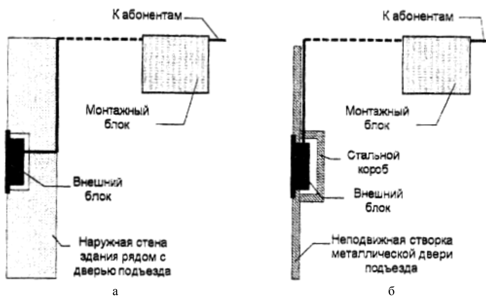
Рисунок 18 - Варианты монтажа блоков подъездного домофона:
